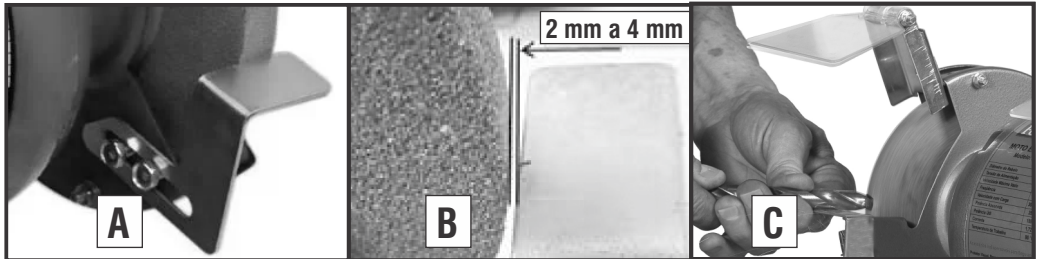
Fig. 4 – Regulagem da mesa de apoio da peça
