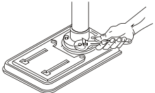
Fig. 1: fixar a coluna na base, alinhado os buracos da coluna com os da base, usando os parafusos (4) 8x20mm.
